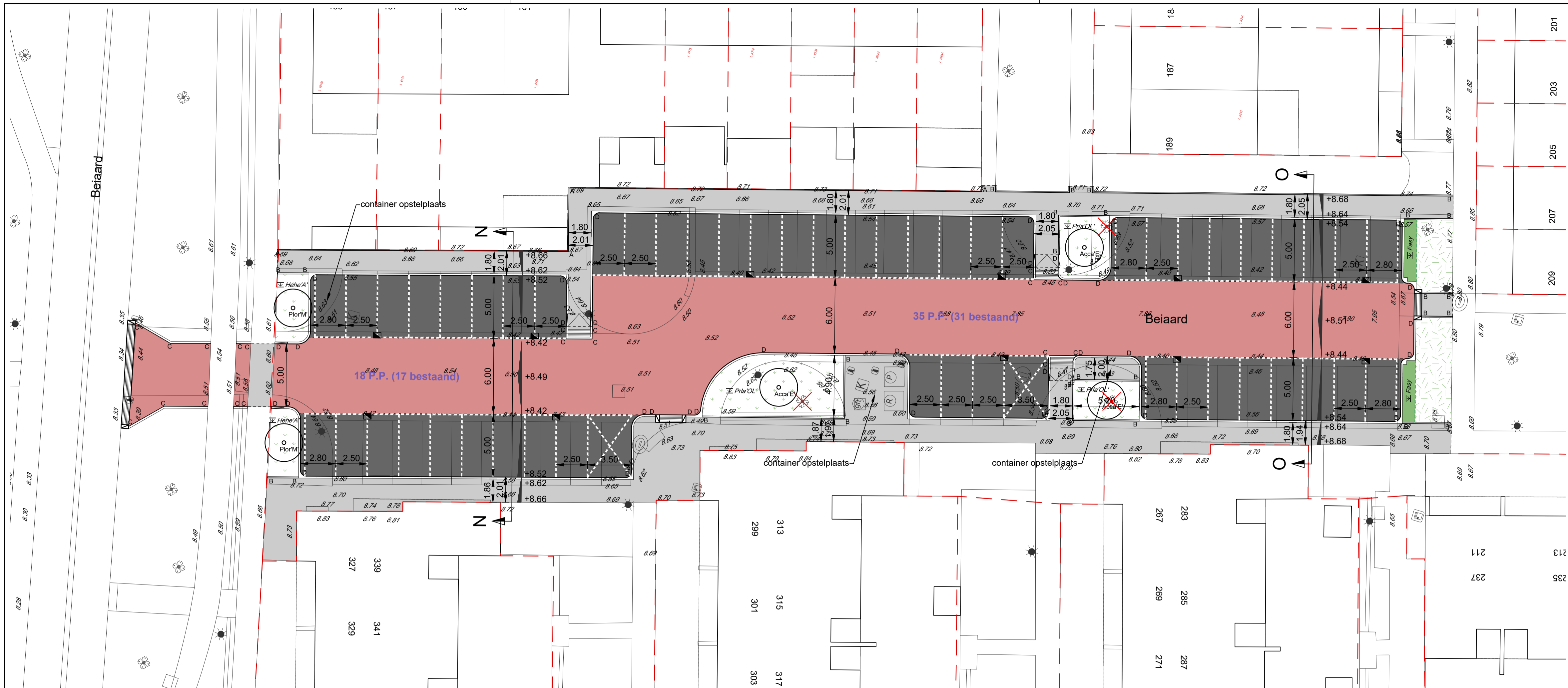
blad 04-1: parkeerhofje 2
