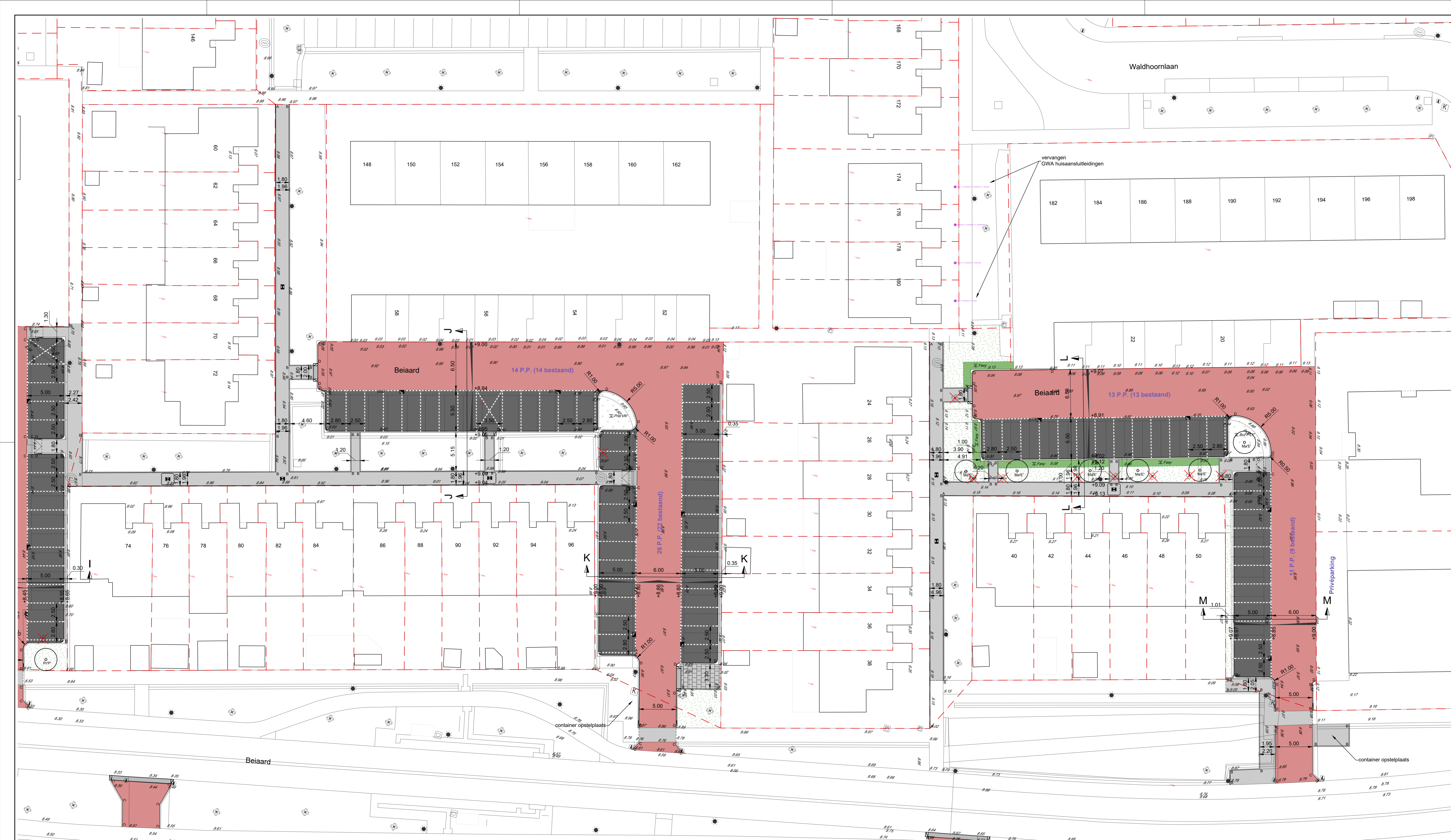
blad 03: parkeerhofje 4 en parkeerhofje 3
